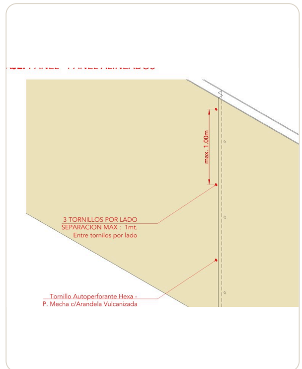
UNIÓN PANEL-PANEL: 3 TORNILLOS POR LADO, MÁX. 1 M
