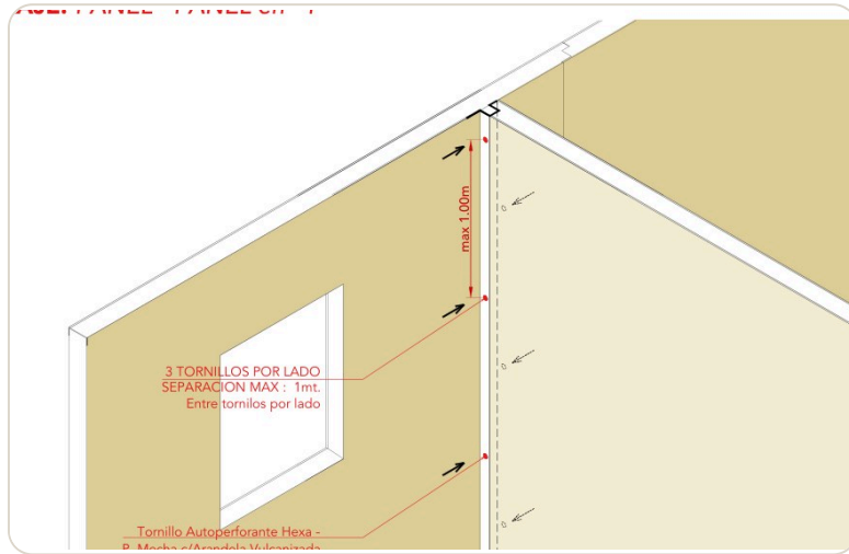
PARED EN "T": PERFIL GALERA VERTICAL
